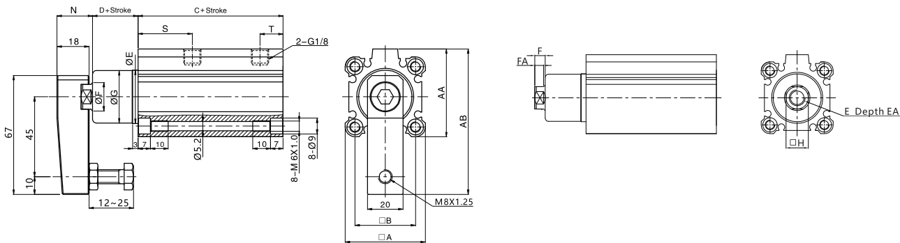
SQKΦ32、Φ40
