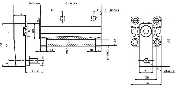
SQKΦ20、Φ25
