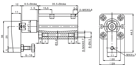
SQKΦ16
